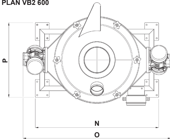
PLAN VB2 600
